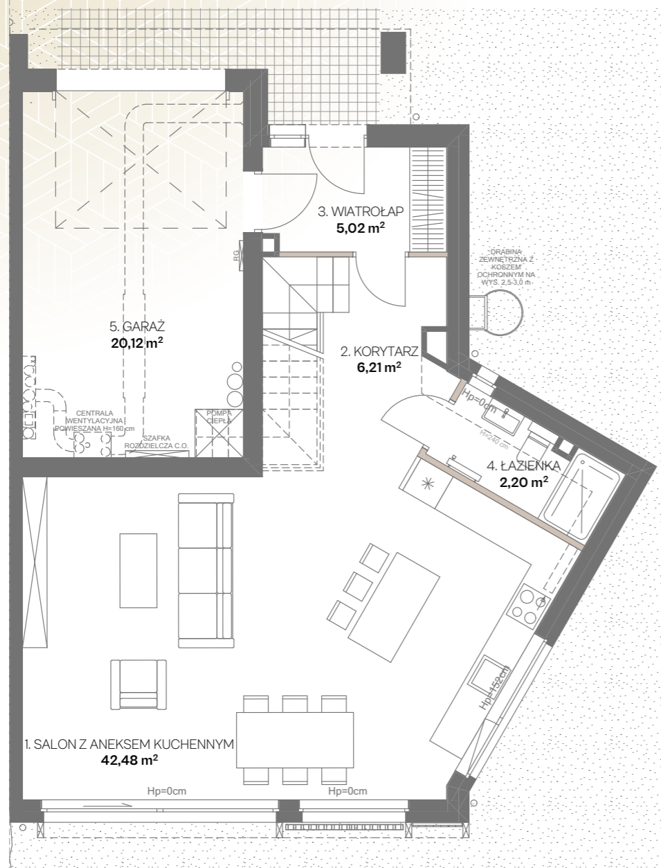
RZUT PARTERU
