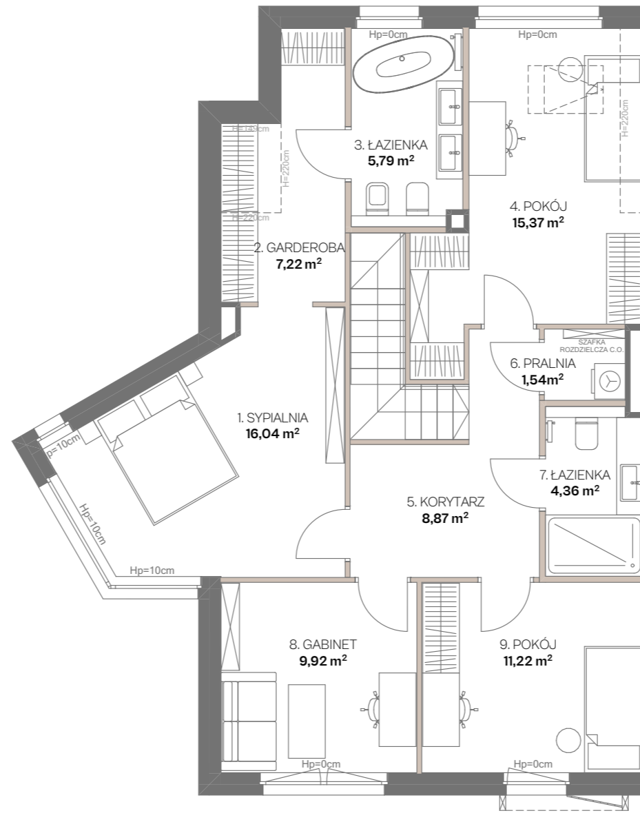
RZUT 1. PIĘTRA
