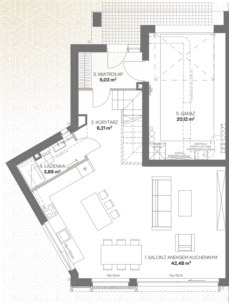
RZUT PARTERU
