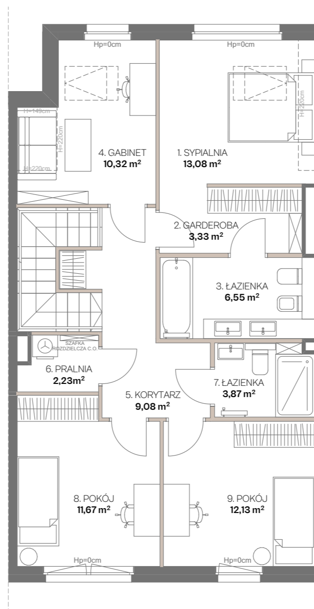
RZUT 1. PIĘTRA
