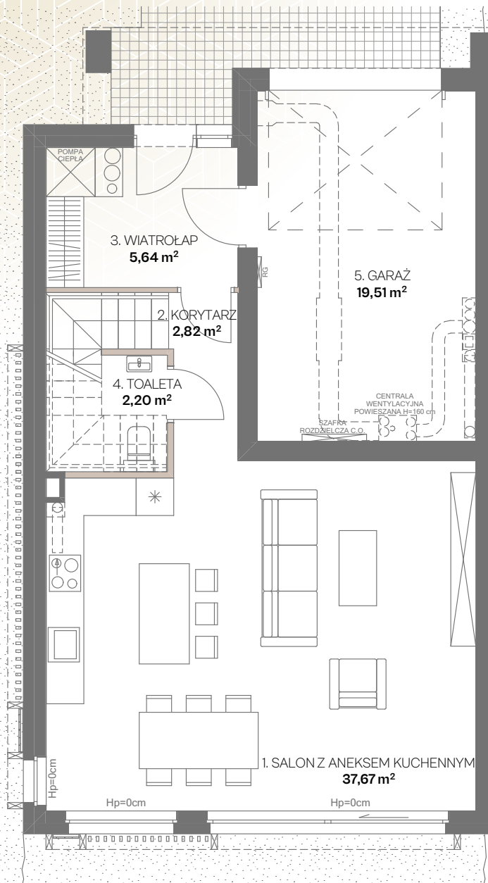
RZUT PARTERU
