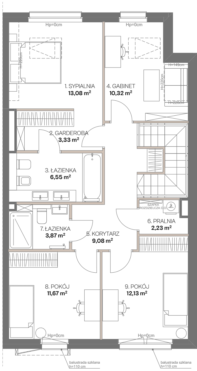
RZUT 1. PIĘTRA
