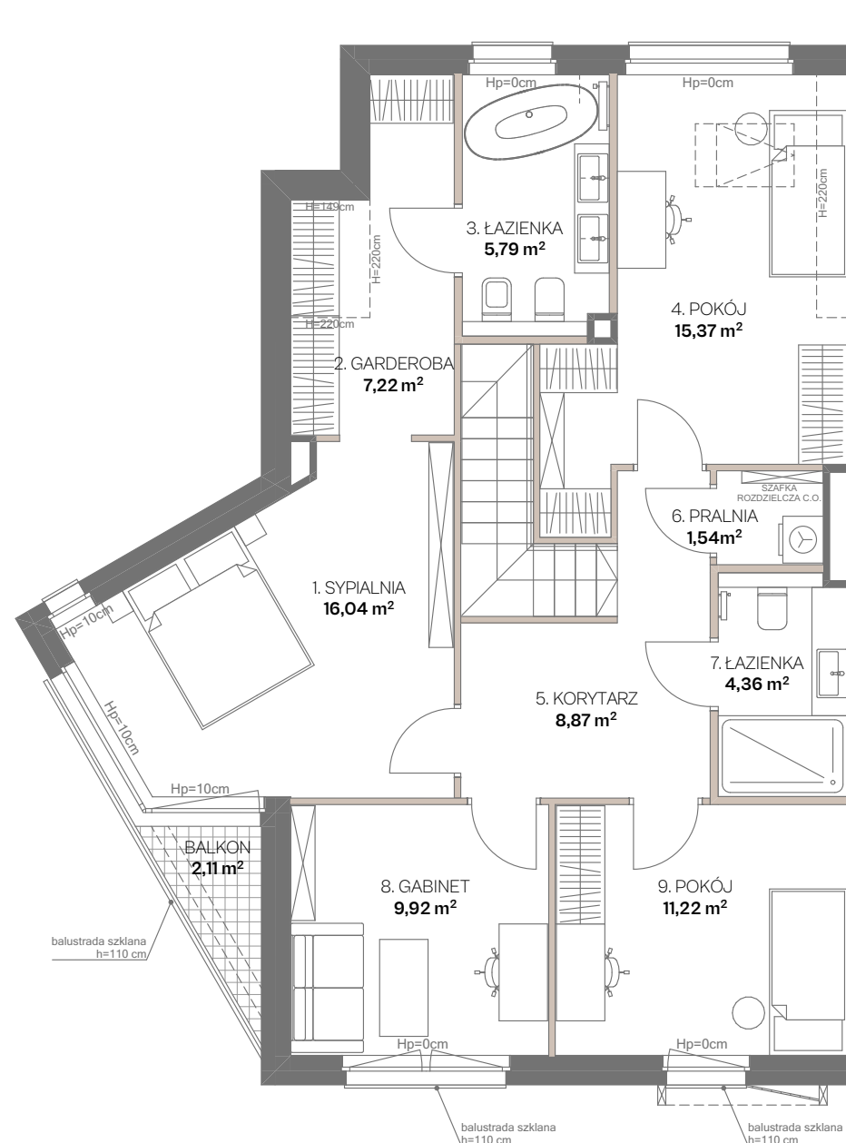
RZUT 1. PIĘTRA
