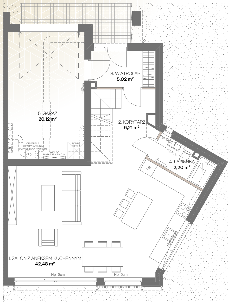
RZUT PARTERU
