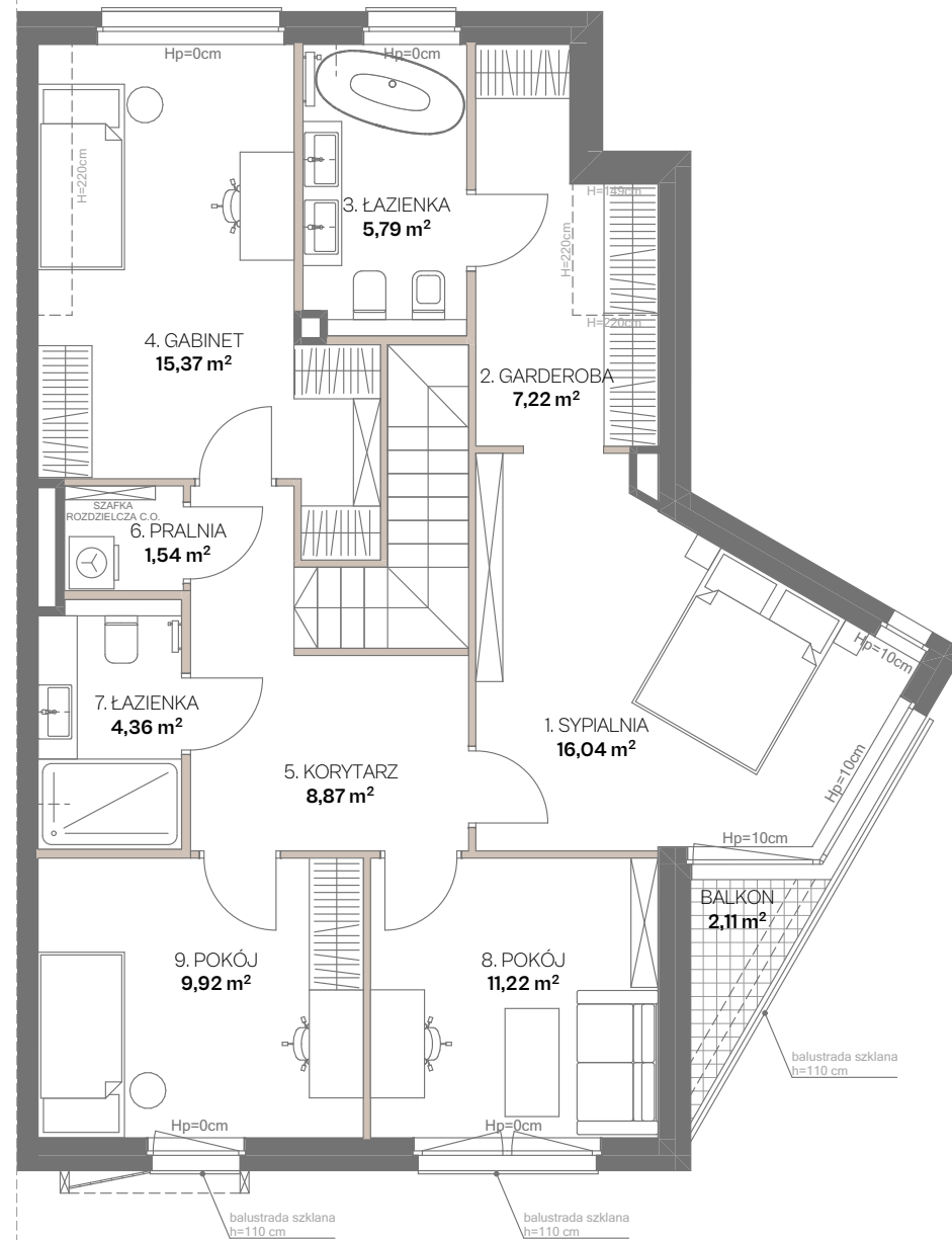
RZUT 1. PIĘTRA
