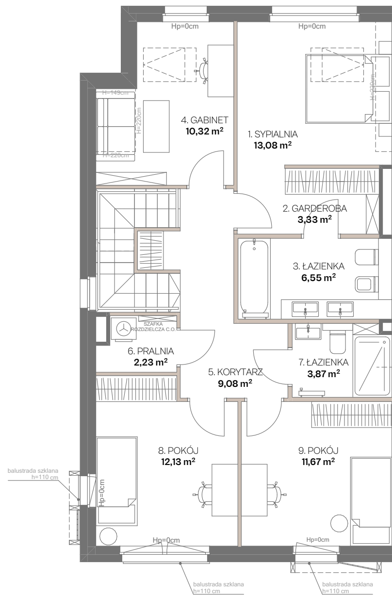
RZUT 1. PIĘTRA
