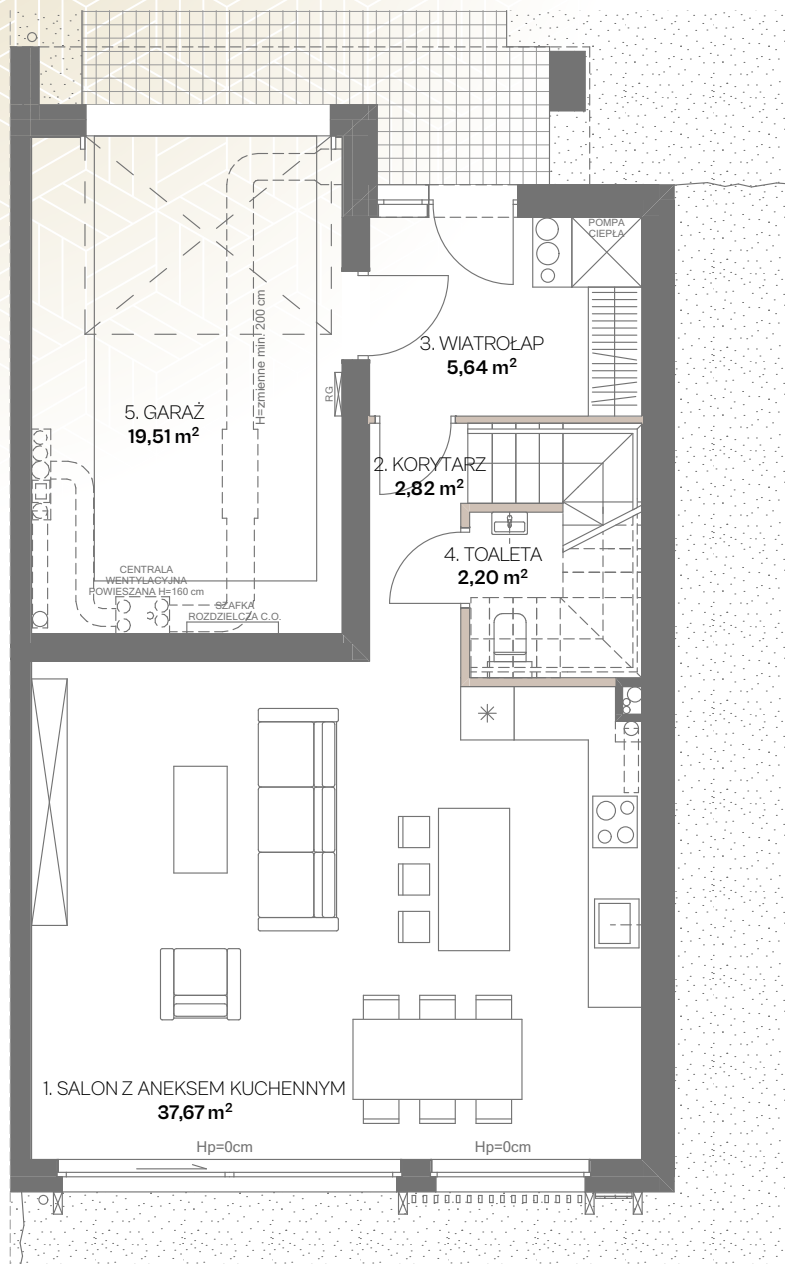
RZUT PARTERU
