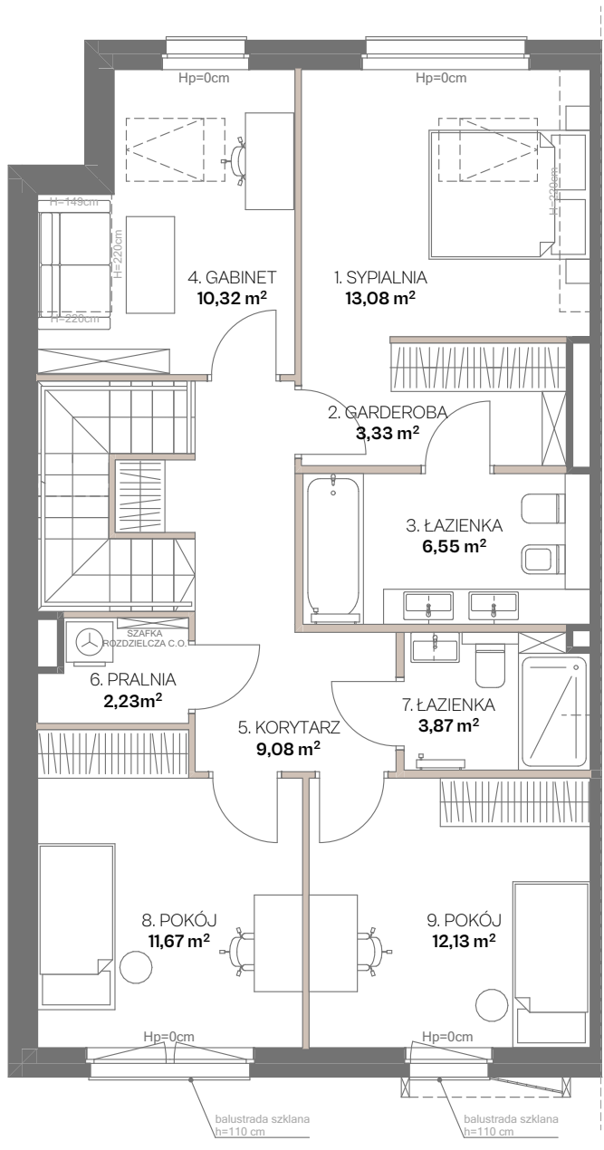
RZUT 1. PIĘTRA
