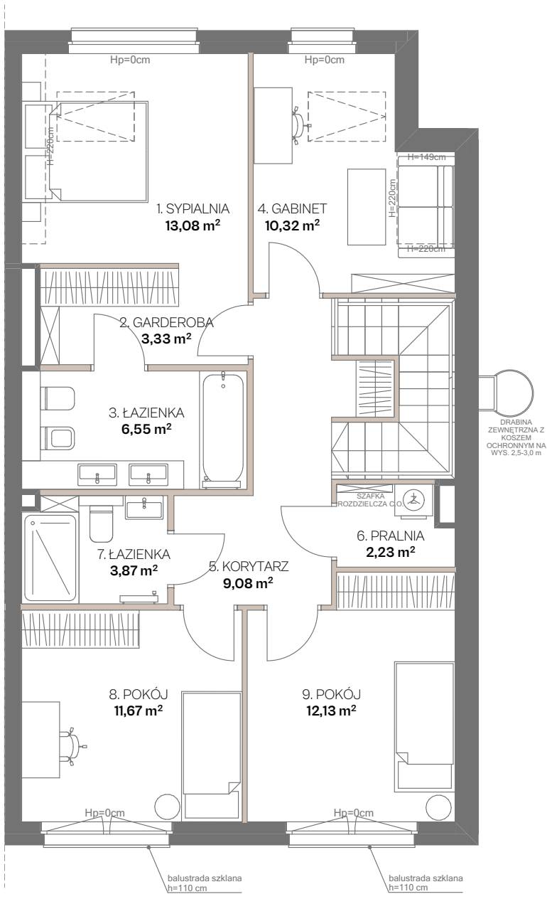
RZUT 1. PIĘTRA
