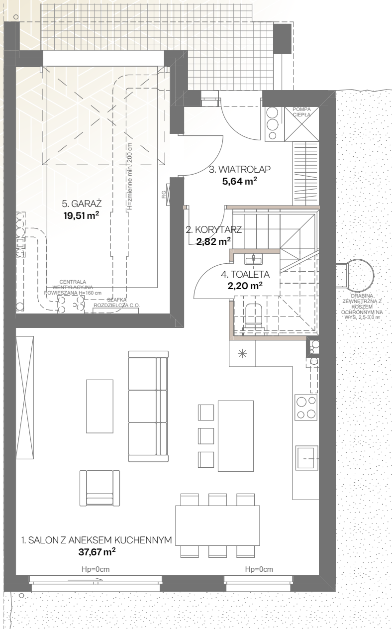
RZUT PARTERU
