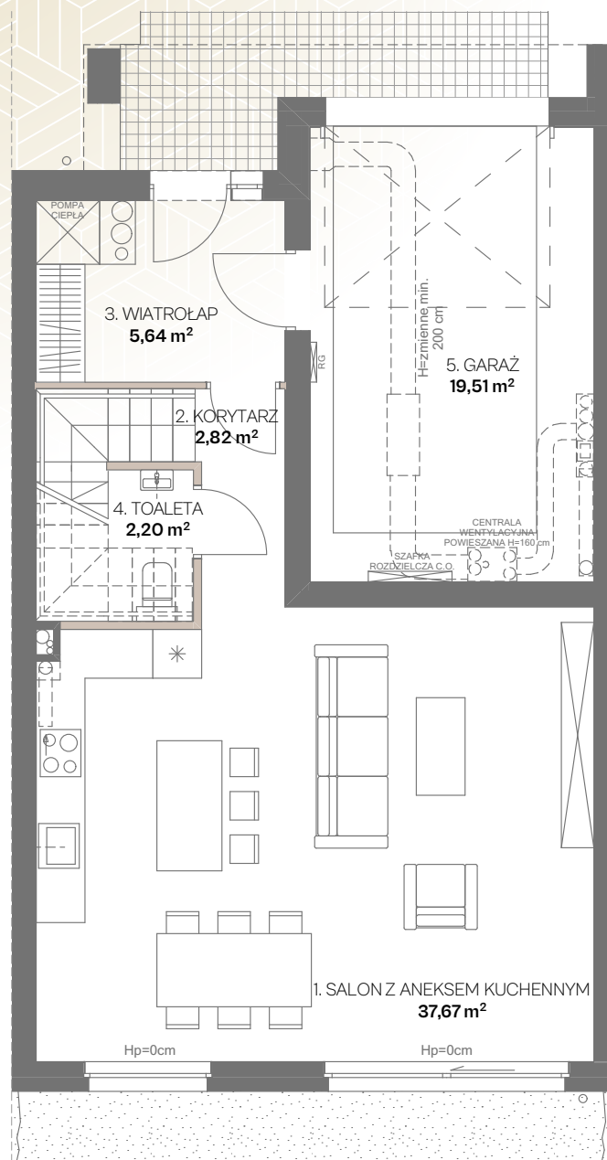
RZUT PARTERU
