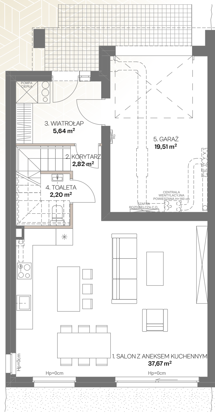
RZUT PARTERU
