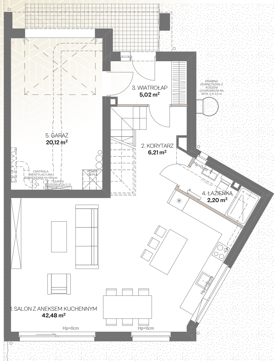
RZUT PARTERU
