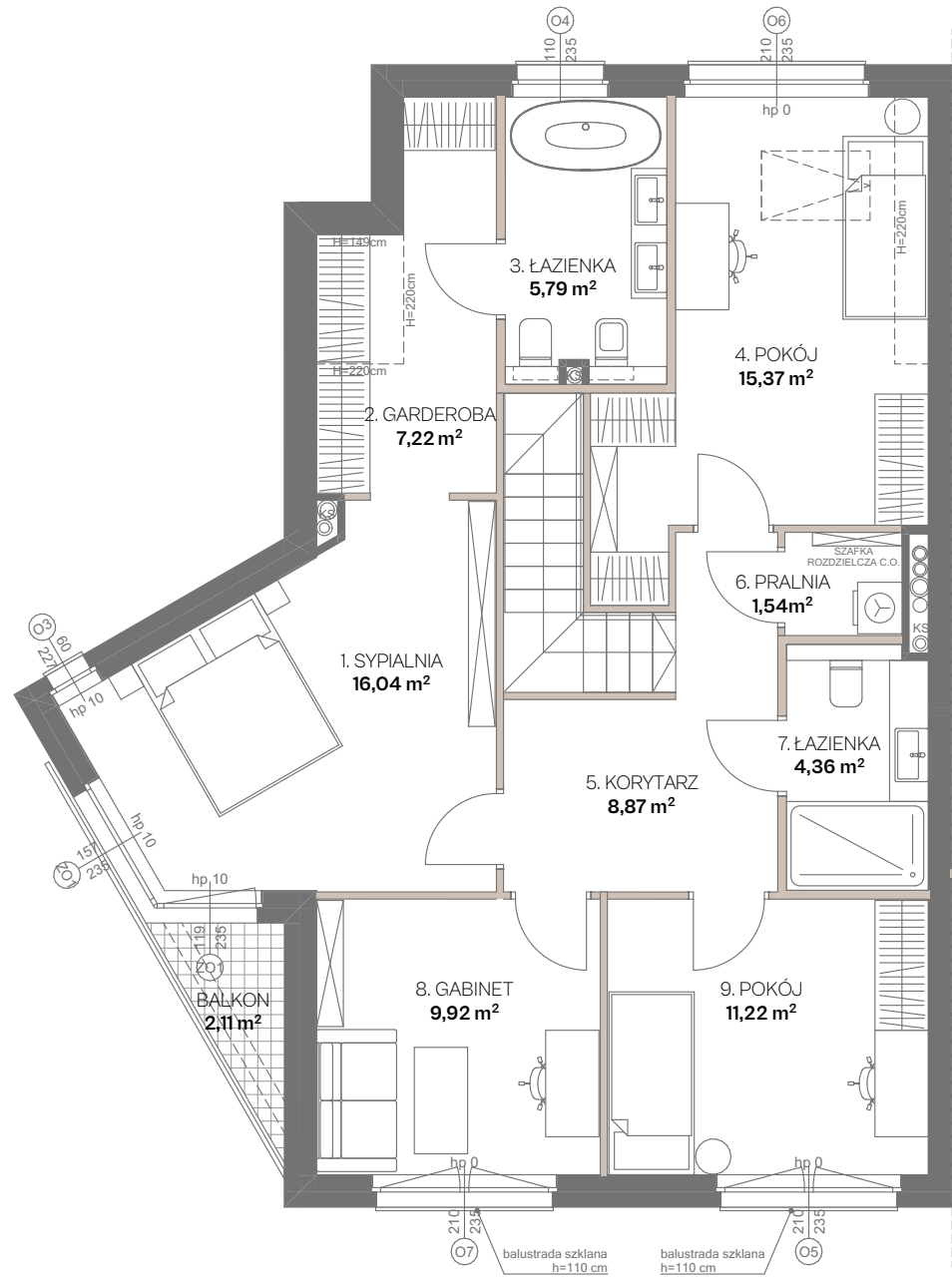
RZUT 1. PIĘTRA
