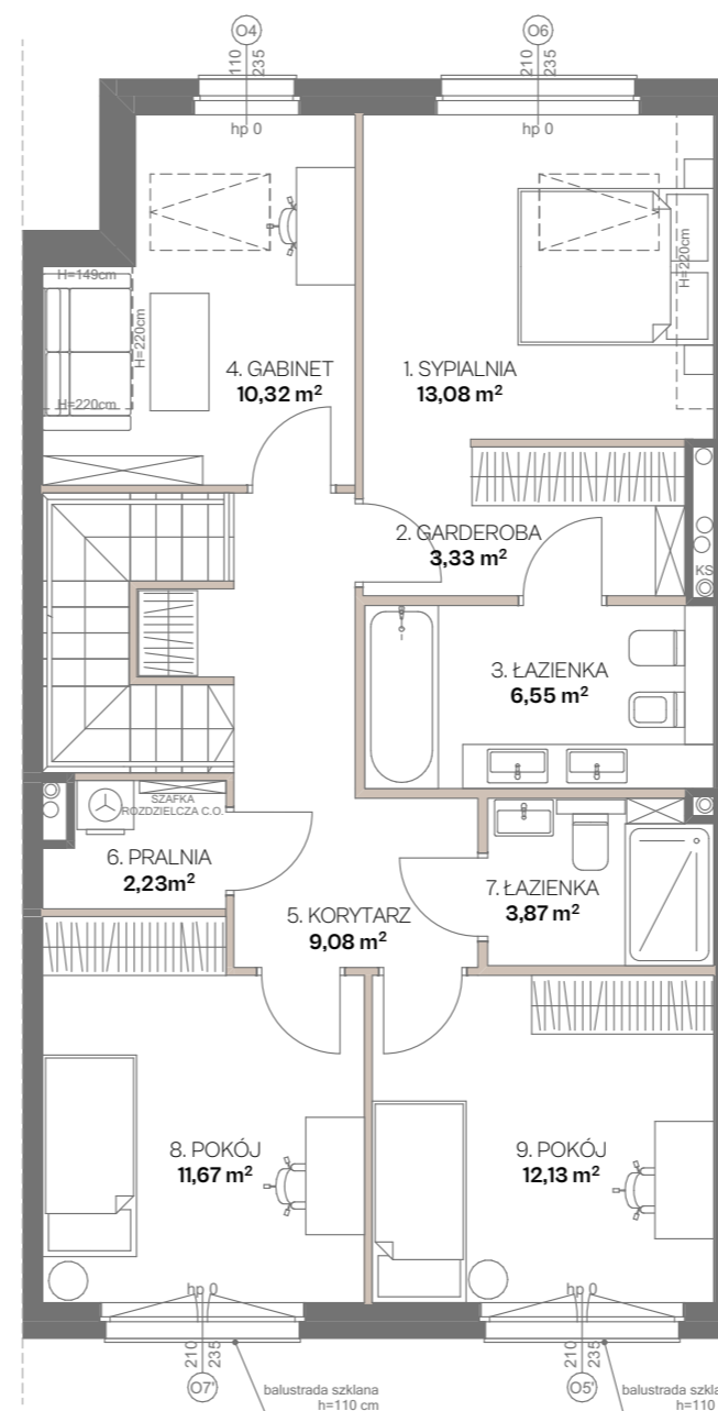
RZUT 1. PIĘTRA
