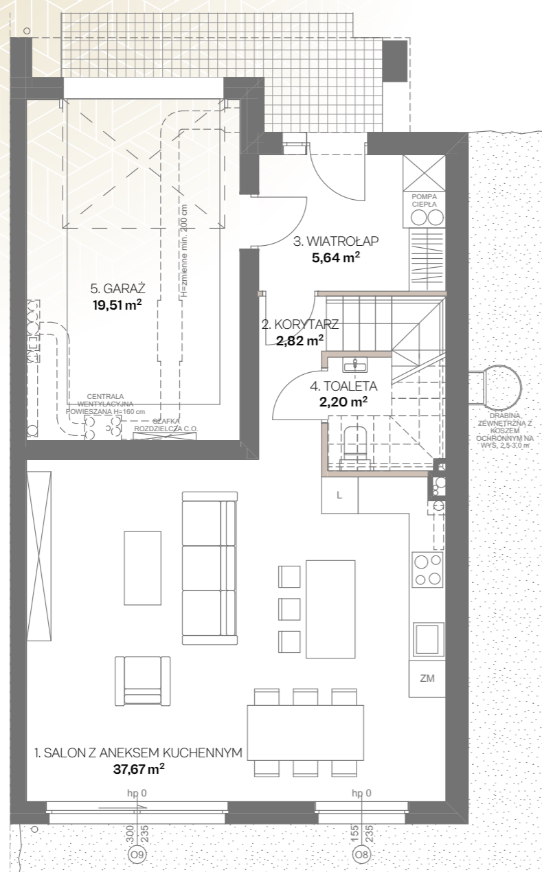
RZUT PARTERU
