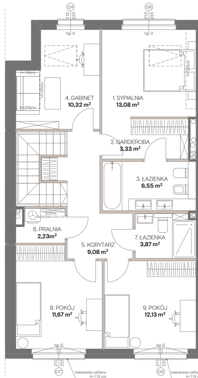
RZUT 1. PIĘTRA
