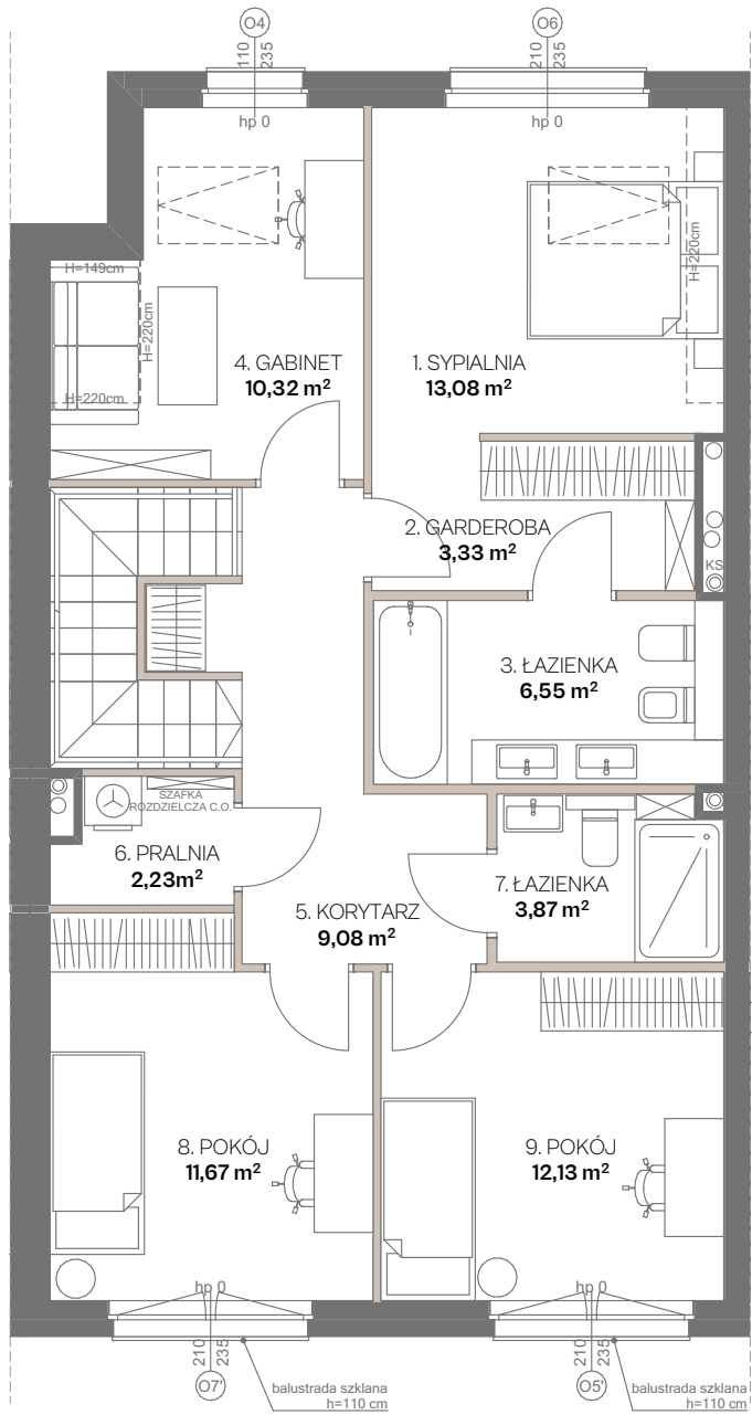
RZUT 1. PIĘTRA
